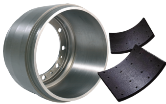
ТОРМОЗНОЙ БАРАБАН 10” PGRT - СЕРИЯ НОМЕР ДЕТАЛИ SCANIA 2378716
